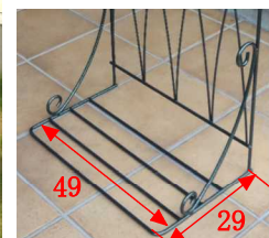
載置部 寸法
